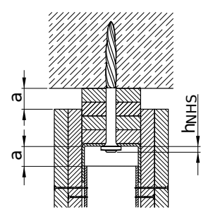
Fixation à tête de déflexion avec bandes de plâtre (en option avec matériau d'étanchéité)
