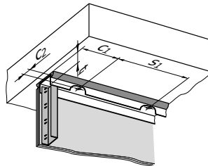
Fijación de carriles con cabezal de desvío (opcional con sellador)
