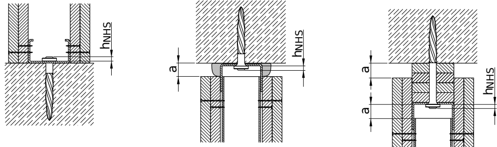
Fijación de perfiles fija Fijación de carriles con cabezal de desvío (opcional con sellador) Fijación del cabezal de desvío con tiras de yeso (opcional con sellador)
