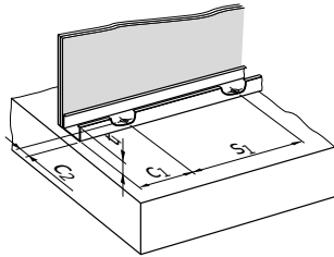
Fijación de perfiles fija
