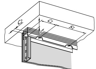
Fissaggio della guida della testa di deviazione con strisce di gesso (opzionale con sigillante)
