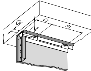
Profilbefestigung Umlenkkopf (optional mit Dichtmasse)
