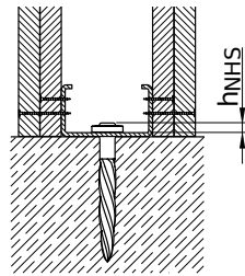
Fixation du rail fixe
