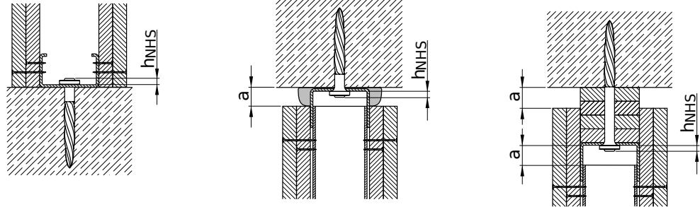
Feste Profilbefestigung Profilbefestigung Umlenkkopf (optional mit Dichtmasse) Umlenkkopfbefestigung mit Gipsstreifen (optional mit Dichtmasse)
