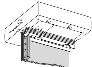
Fixation de rails à tête de déflexion avec bandes de plâtre (en option avec matériau d'étanchéité)
